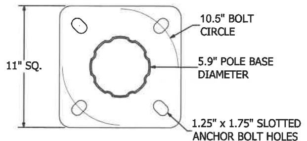
VIEW A-A
